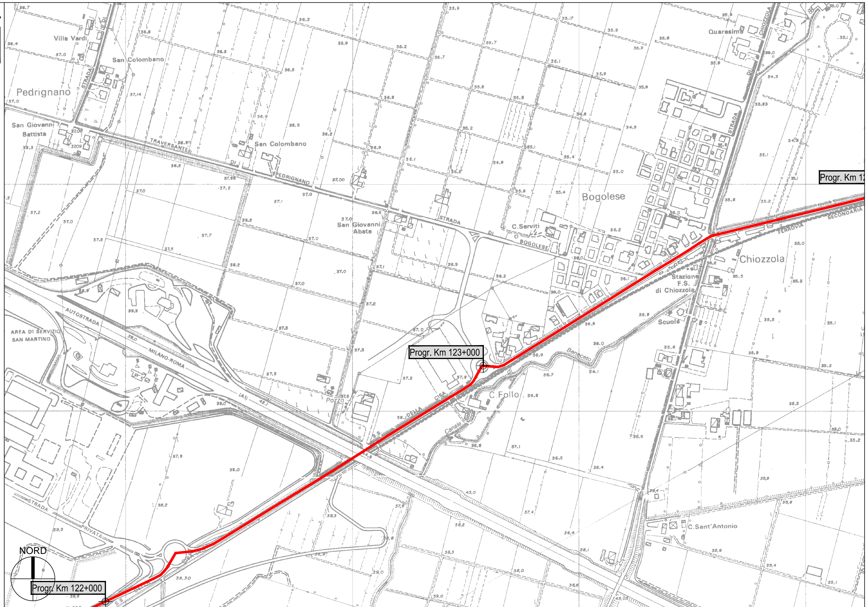
S.P. 62R della Cisa - Sviluppo chilometrico 8+137 km
