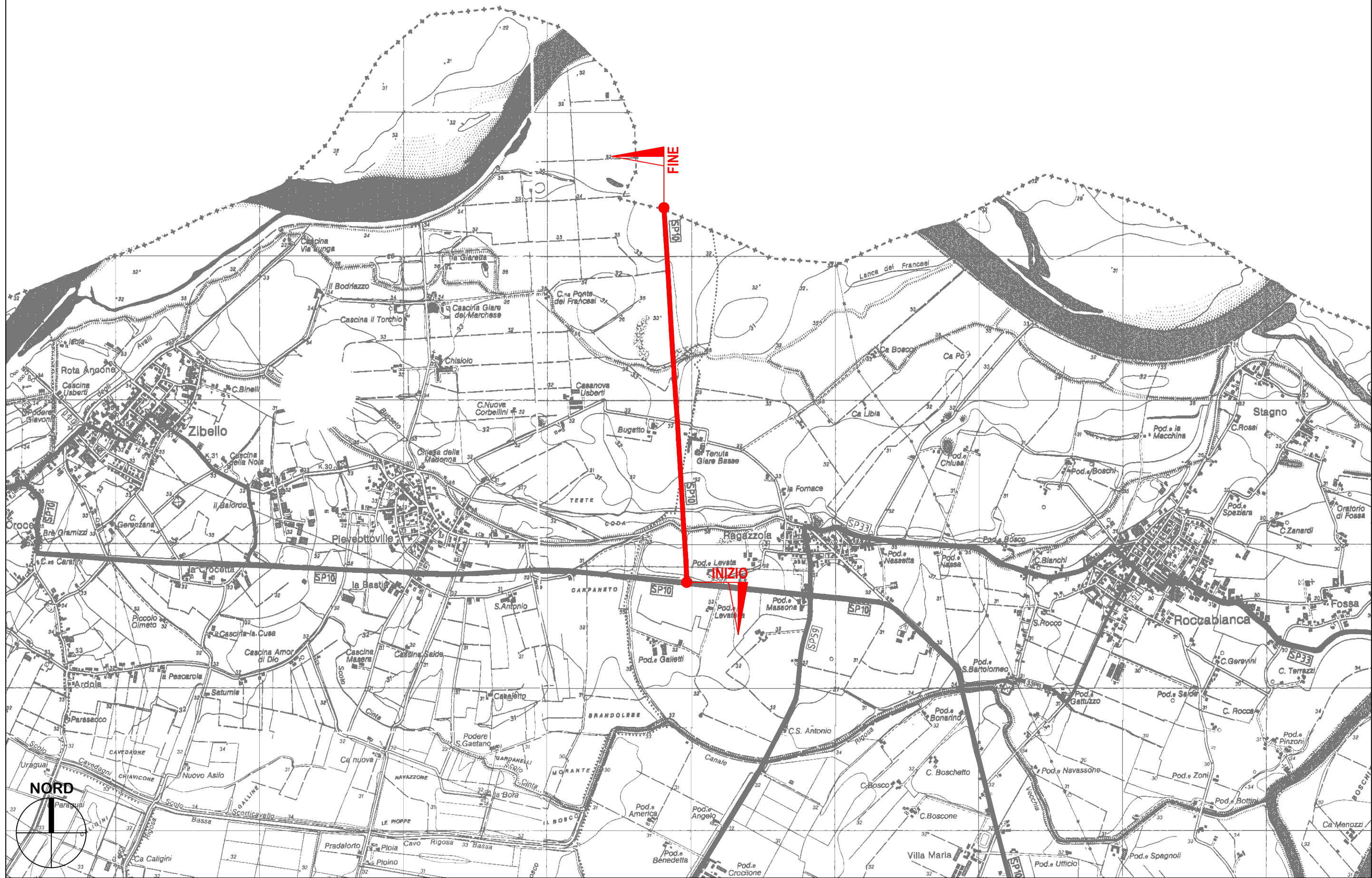
S.P. 10 del Nuovo ponte sul Po - Sviluppo chilometrico 2+610 km
