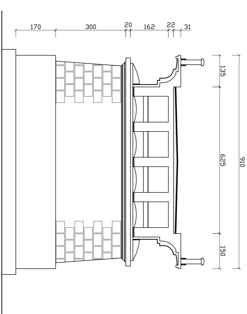
Sezione su Appoggio di testa della travata
