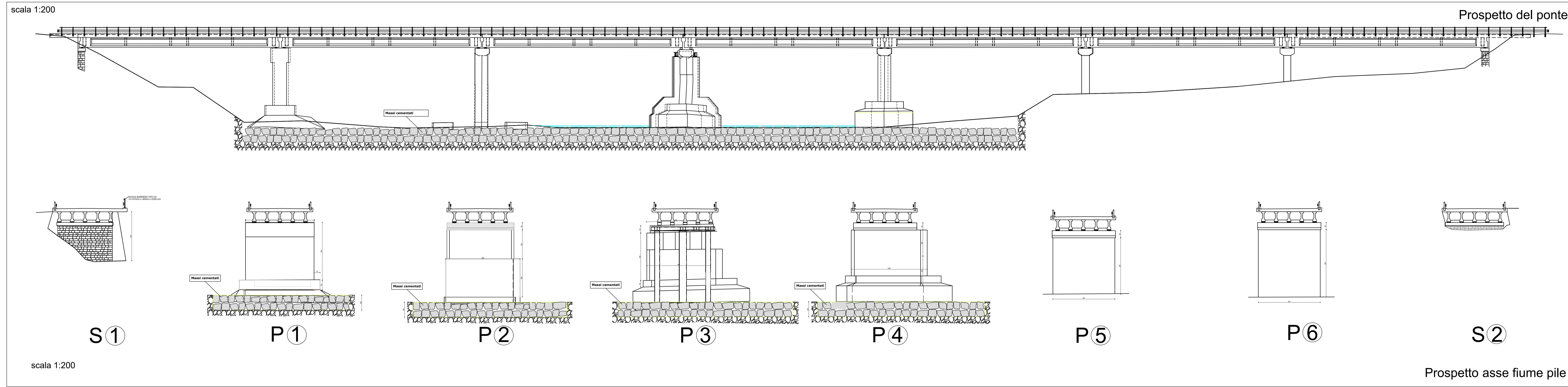
Pianta filo travi del ponte
